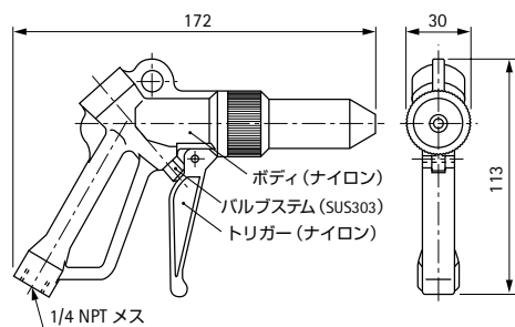
ガス フィルター ガン 本体
