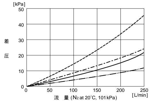
--- 6段 INLET 0.206 MPa -.- 12段 INLET 0.206 MPa — 6段 INLET 0.618 MPa -.- 12段 INLET 0.618 MPa
