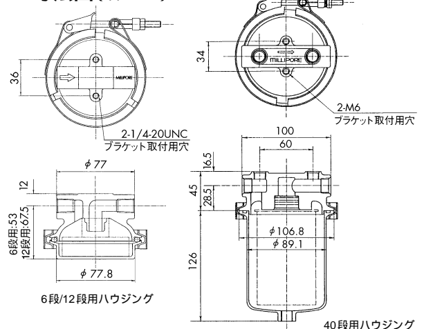
40段用ハウジング
